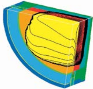
Расчетная модель установки
