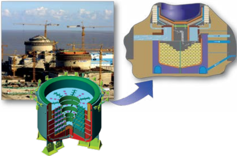
Устройство локализации расплава активной зоны на Тяньваньской АЭС
