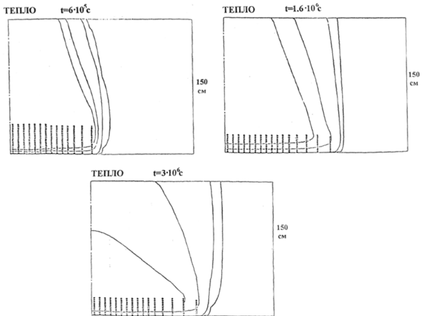
Расчетное моделирование растекания цилиндрического фрагмента топлива по охлаждаемой плите теплообменника
