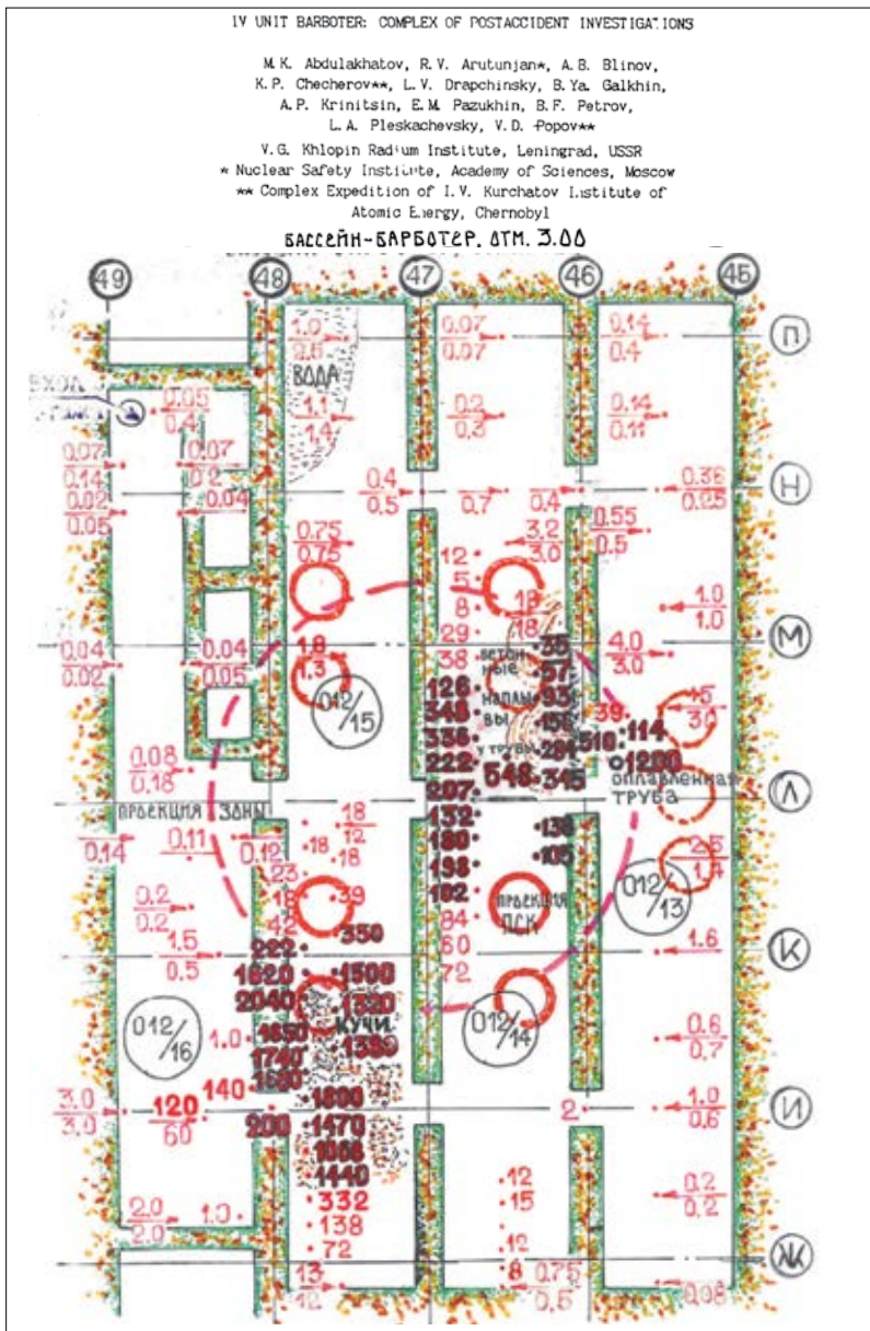
Док. 22. Схема распределения мощности дозы в бассейне-барботёре. Впервые представлена на первой международной рабочей группе по тяжёлым авариям в Дагомысе, 1989 г.
